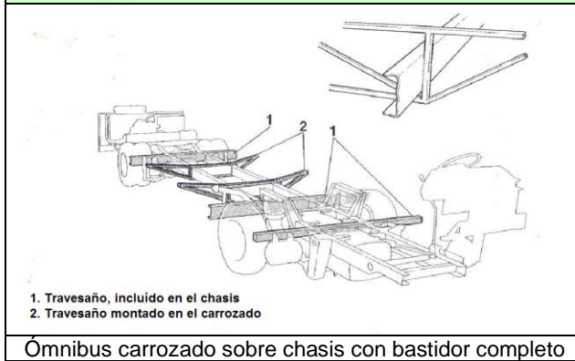
Figura II.1 : Ómnibus Convencional
